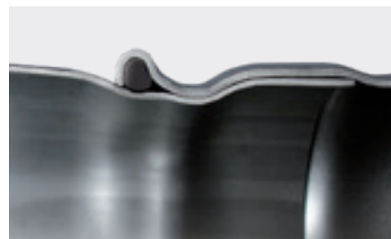
Mekaniskt stabil och hydrauliskt läckagefri: pressfogen.
