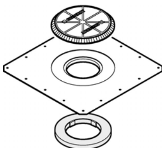
Pluvia påsvetsningsplatta
